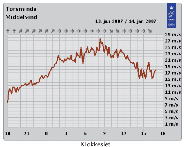
Middelvind – data fra Torsminde fra d. 13.-14. januar, 2007. (Grafik: gengivet med tilladelse fra DMI)
